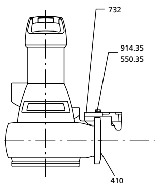
Рис. 11: Монтаж держателя
