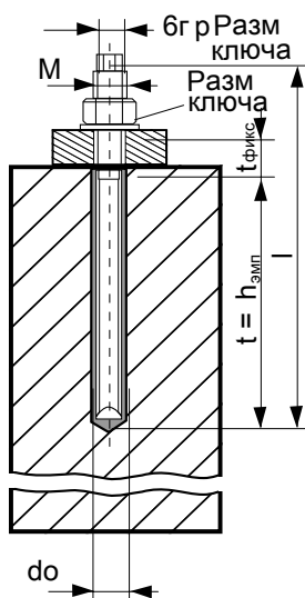
Рис. 7: Размеры
