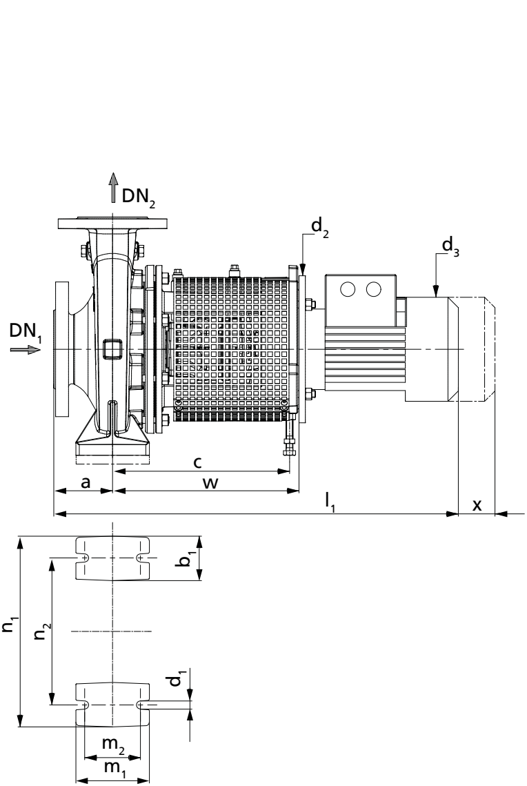
Габаритные размеры
