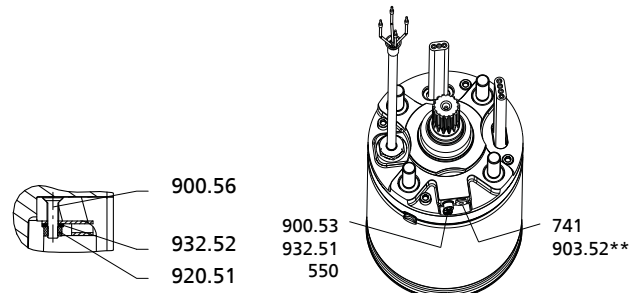
Крепление заземления
